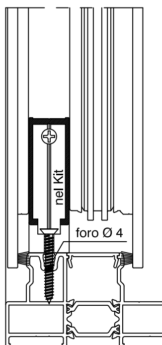
TELAIO TT170.04
