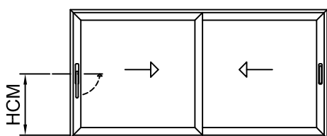
PROSPETTO INTERNO
