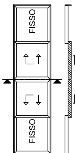
SCHEMA C (prospetto interno)
