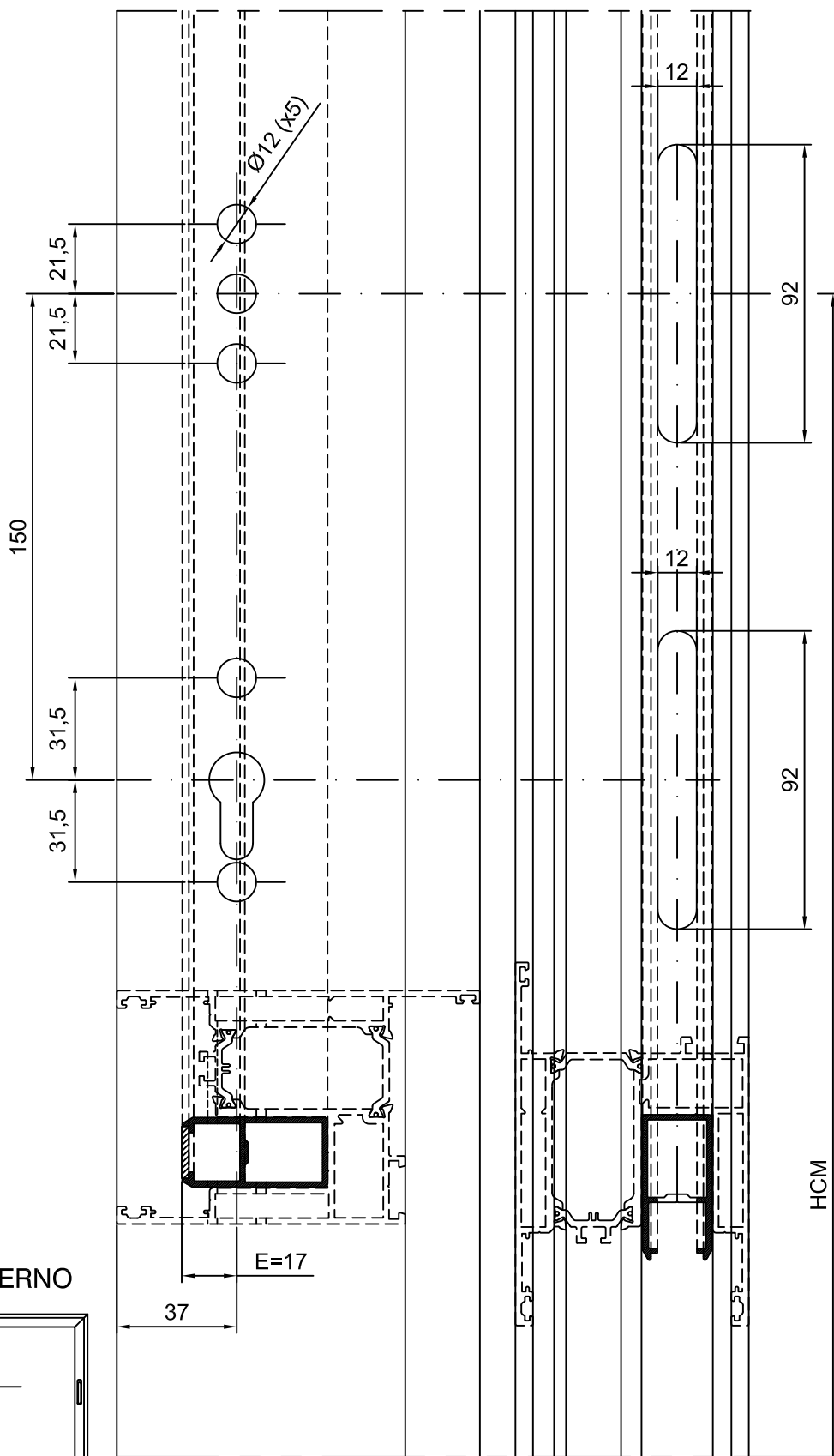
VISTA FRONTALE INTERNA
